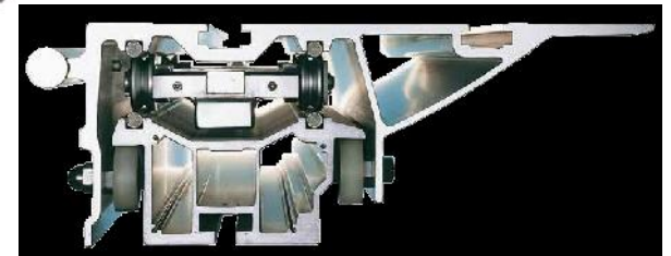
Profil aluminium anodisé de structure tubulaire assurant une grande rigidité de la table. Déplacement assuré par des galets spécialement profilés sur des guides acier cimentés
